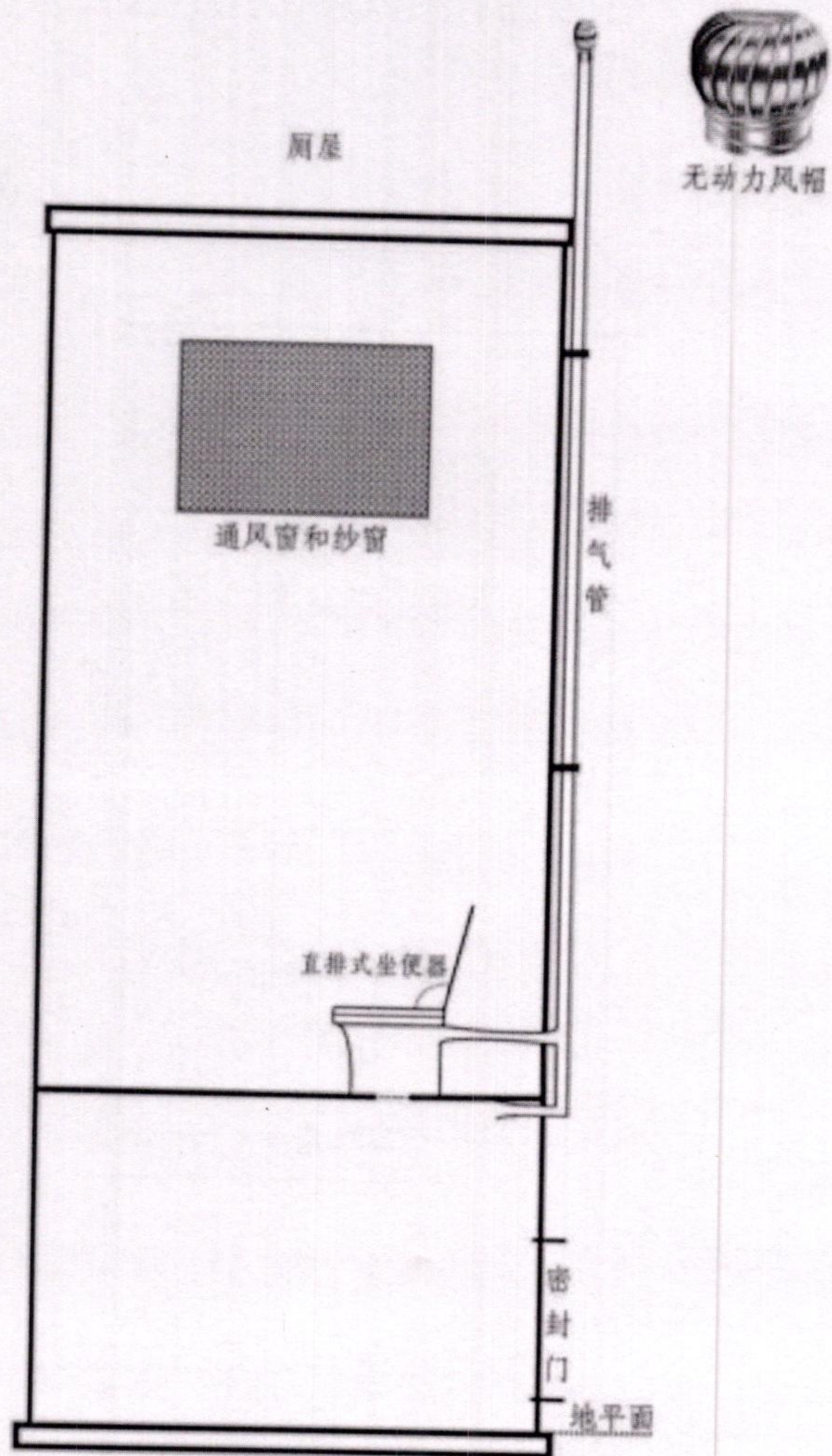
2-农村积肥式户用卫生旱厕构造示意图
