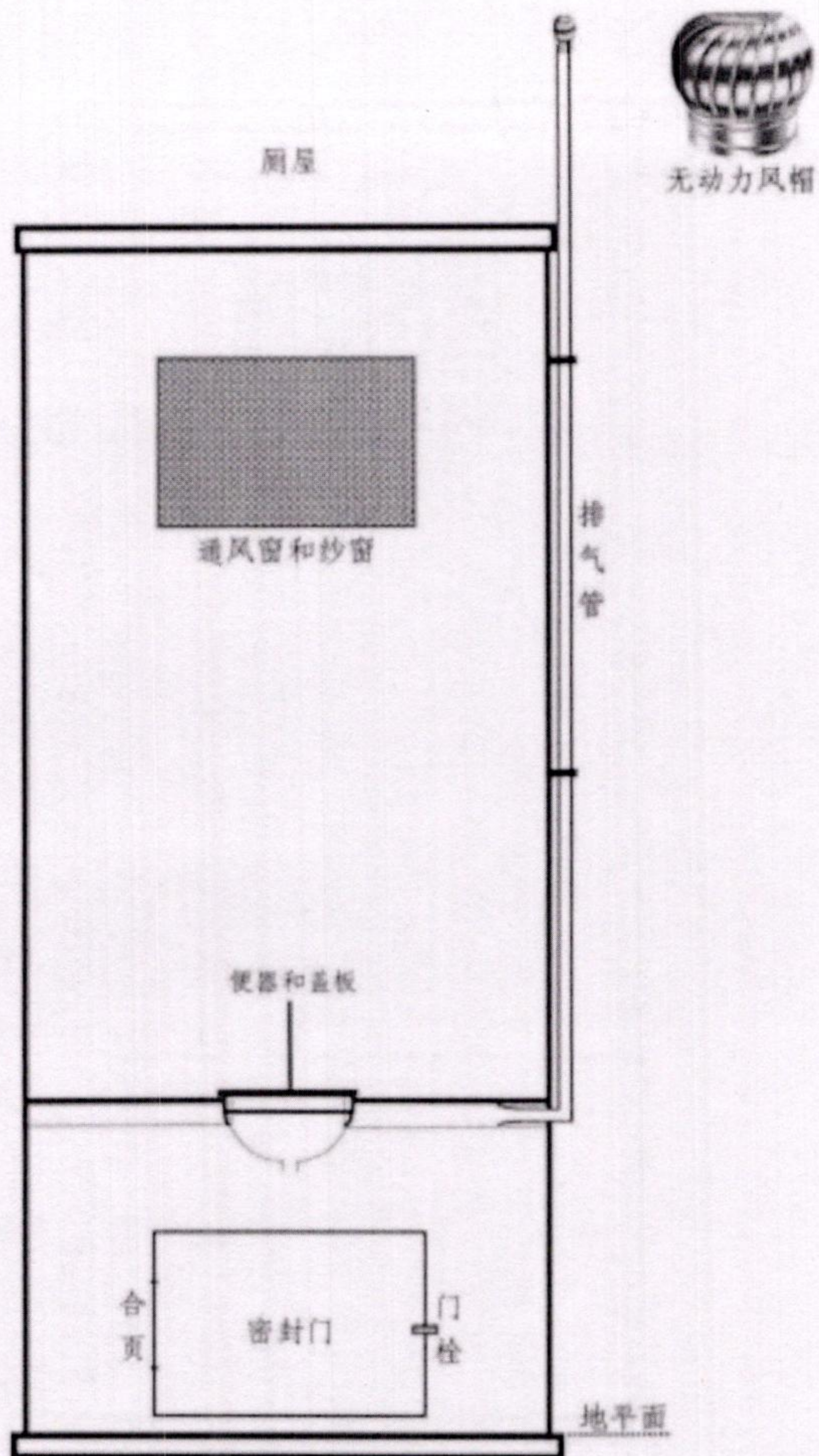
1-农村积肥式户用卫生旱厕构造示意图
